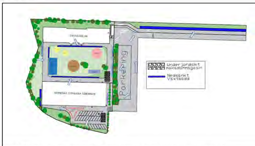
Figur 6-3. Föreslagen dagvattenhantering. Figuren redovisar enbart lösningarnas anläggningsyta.
