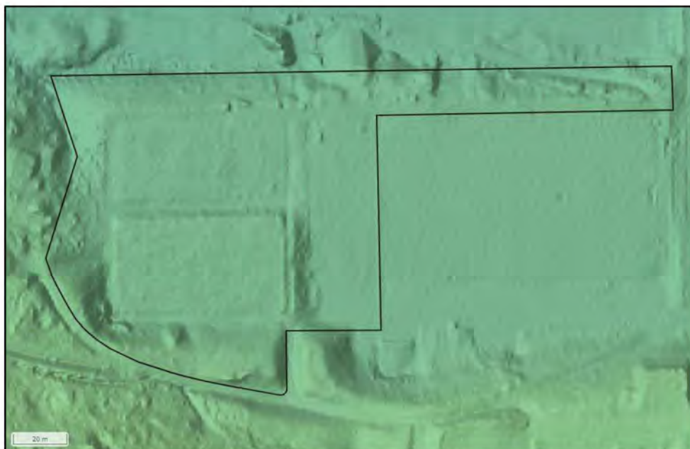
Figur 32. Topografiskarta. Plangränsen markerad med svart linje. (Scalgo Live, 2023)
