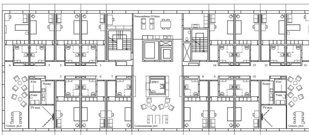
Våningsplan (ritad av Kolman Boye Arkitekter AB)
