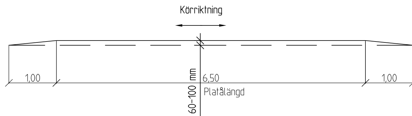
Platågupp - profil Gator utan busstrafik 1:50
