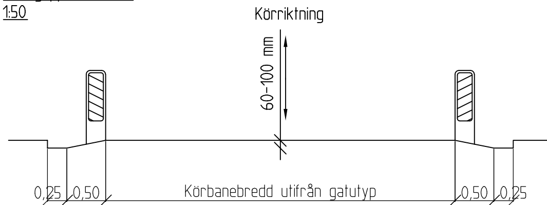
Platågupp - profil Gator utan busstrafik 1:50
